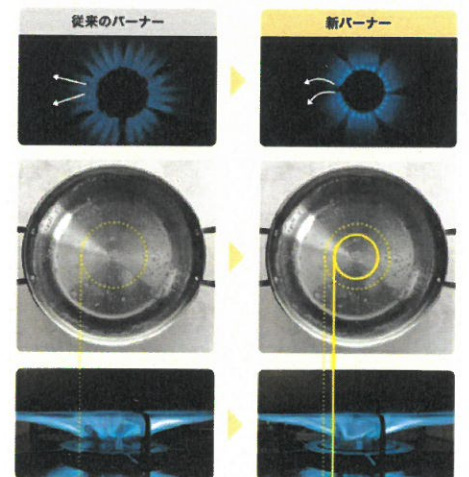
小径化された新バーナーは、炎と鍋が接する距離が狭く、効率よく加熱できます。
